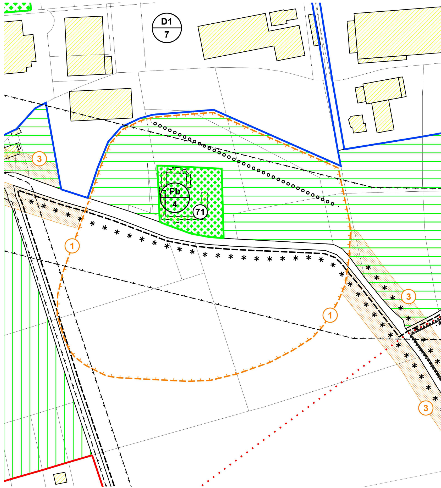
Estratto P.R.G. Vigente - Scala 1:2000
